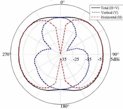
UMTS ( f_c = 2045\text{MHz} )
